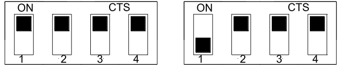
图 6-13 JTY-GXF-GST2D 模组地址设置
