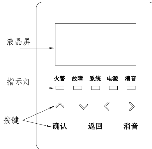
图 3-1 探测器显示及操作面板示意图
