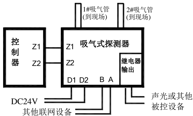
图6-9 接线示意图
